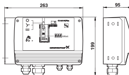
Fig. 18 Dimensions
